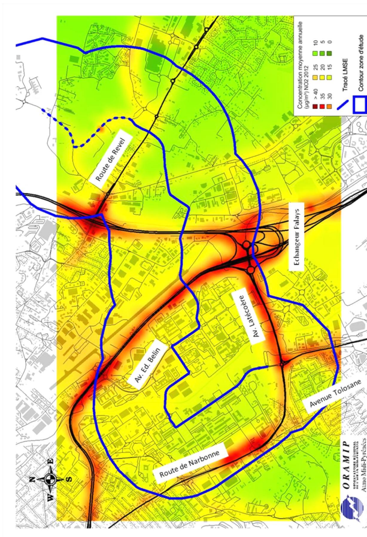
Carte 3 : Cartographie des concentrations moyennes annuelles modélisées en NO 2 , le long de la LMSE (dans la zone d'étude)
