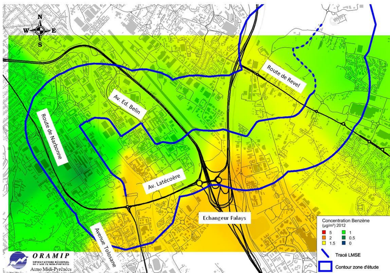
Carte 4 : Cartographie des concentrations moyennes annuelles modélisées en Benzène, le long de la LMSE (zone d'étude)
