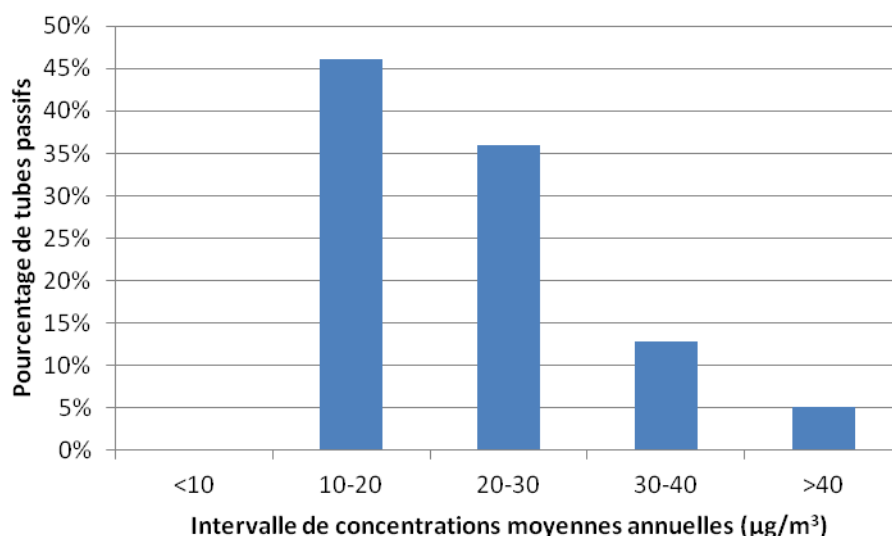
Graphique: Répartition des tubes passifs en fonction des intervalles de concentration en NO 2 pour l'année 2012
