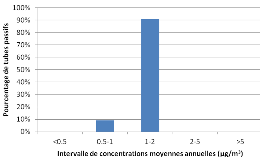
Graphique: Répartition des tubes passifs en fonction des intervalles de concentration en benzène pour la période de mesure
