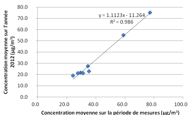
Graphique: Droite de régression linéaire entre les concentrations NO 2 mesurées sur la période et sur l'année des stations toulousaines
