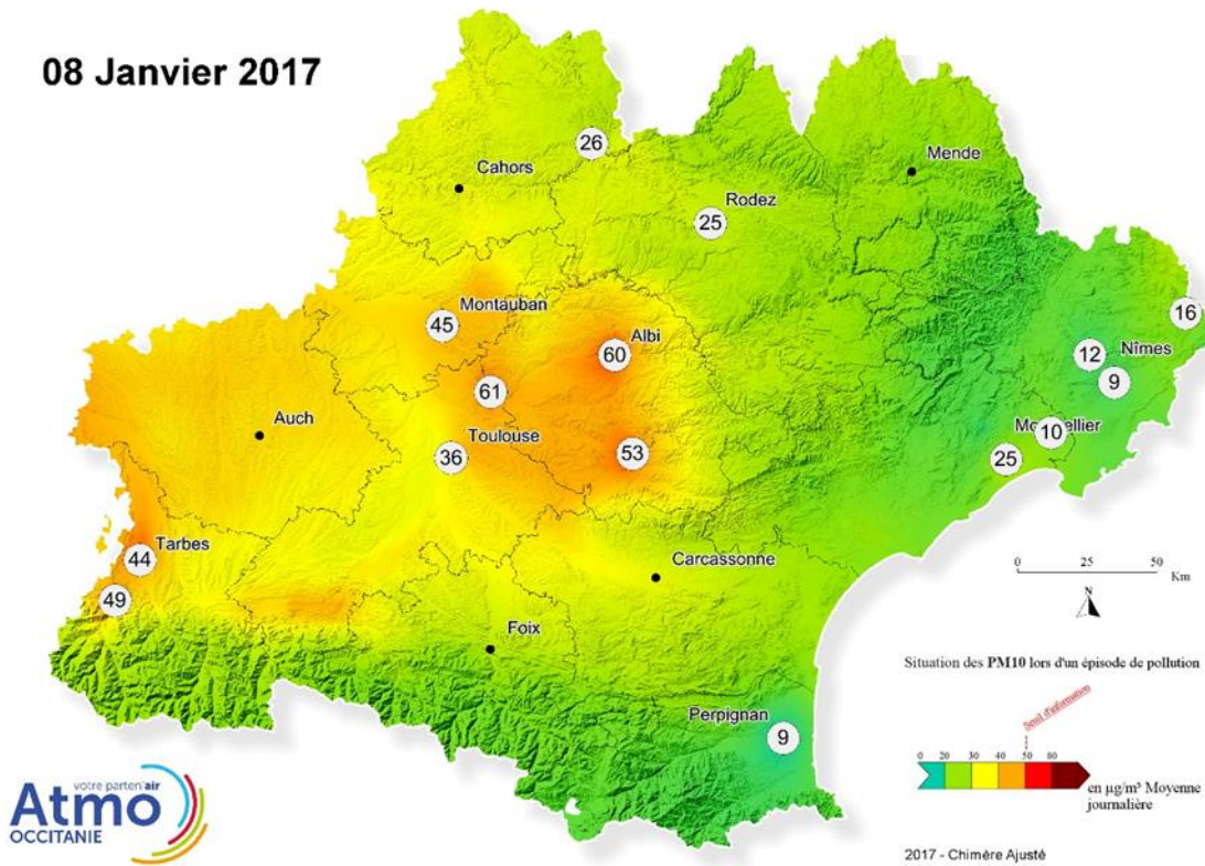
Concentration moyenne journalière du 8 janvier 2017
