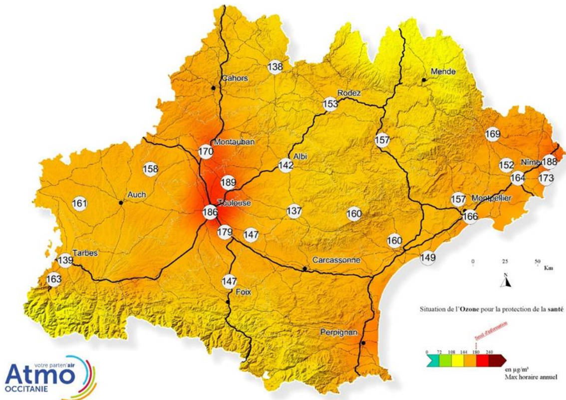
Concentration maximale horaire- année 2017
