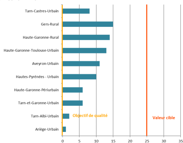
Nombre de jours de concentrations supérieures à 120 \mu\text{g}/\text{m}^3 en moyenne sur 8 heures
