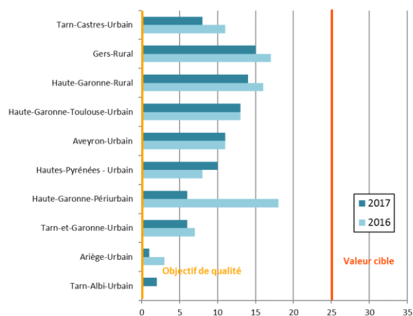
Nombre de jours de concentrations supérieures à 120 \mu\text{g}/\text{m}^3 en moyenne sur 8 heures en 2016 et 2017
