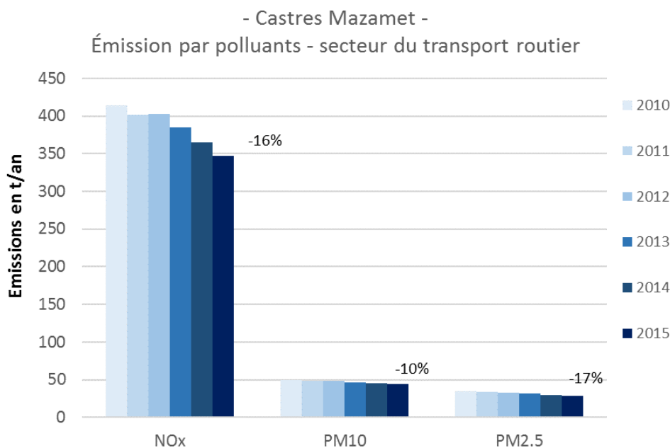
Graphie 13 : Évolution des émissions de polluants atmosphériques secteur TRANSPORT ROUTIER - Castres Mazamet- avec évolution 2010/2015
