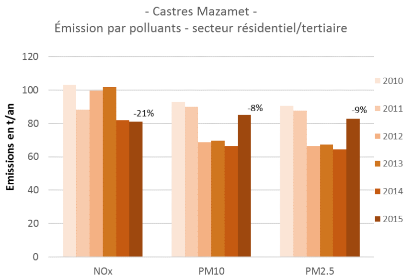
Graphe 14 : Évolution des émissions de polluants atmosphériques secteur RESIDENTIEL/TERTIAIRE - Castres Mazamet- avec évolution 2010/2015
