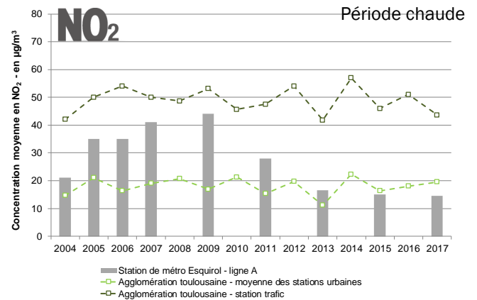
Graph 22 : Évolution des concentrations moyennes en DIOXYDE D'AZOTE sur la période chaude mesurées dans la station de métro ESQUIROL depuis 2007 et comparaison avec les concentrations rencontrées dans l'air ambiant extérieur.
