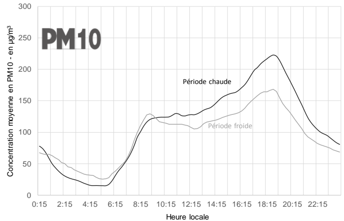
Graphe 5 : Comparaison des niveaux en PARTICULES PM10 mesurés sur une journée moyenne en PÉRIODE CHAUDE et en PÉRIODE FROIDE - station de métro ESQUIROL.
