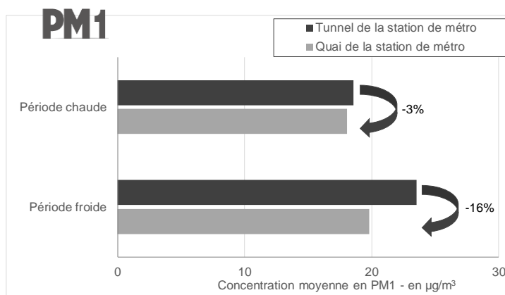
Graphe 17 : Niveaux en PARTICULES PM1 mesurés sur le QUAI dans le TUNNEL - station de métro ESQUIROL
