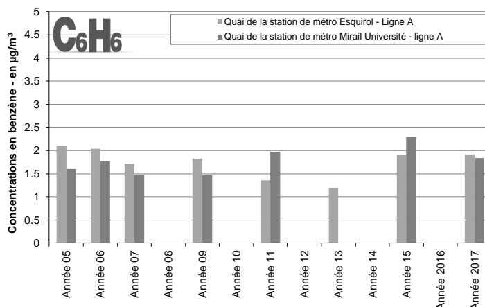
Graph 25 : Évolution des concentrations en BENZÈNE en moyenne sur les deux périodes mesurées dans les stations de métro de la ligne A depuis 2005.
