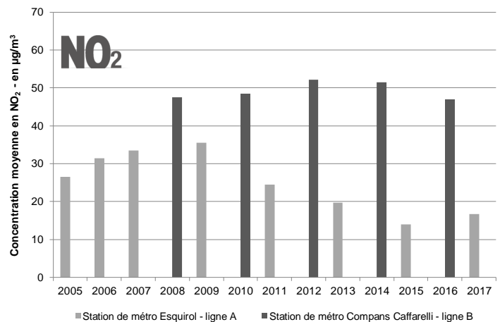
Graph 23 : Évolution des concentrations en DIOXYDE D'AZOTE en moyenne sur les deux périodes mesurées dans une station de métro de la ligne A depuis 2005 et comparaison avec les concentrations mesurées sur la ligne B.
