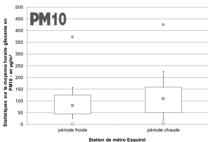
Graphe 8 : Répartition des concentrations horaires en PARTICULES PM10 mesurées dans la station de métro ESQUIROL.
