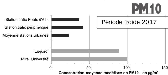
Graphe 3 : Concentration moyenne en PM10 dans les stations de métro et comparaison aux concentrations mesurées dans l'air ambiant extérieur - période froide 2017
