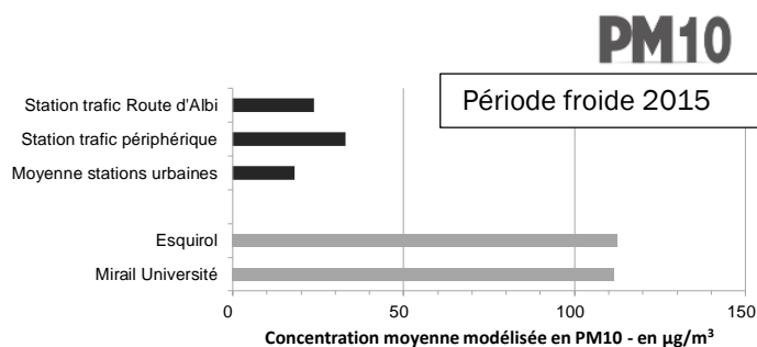
Graphe 2 : Concentration moyenne en PM10 dans les stations de métro et comparaison aux concentrations mesurées dans l'air ambiant extérieur - période froide 2015
