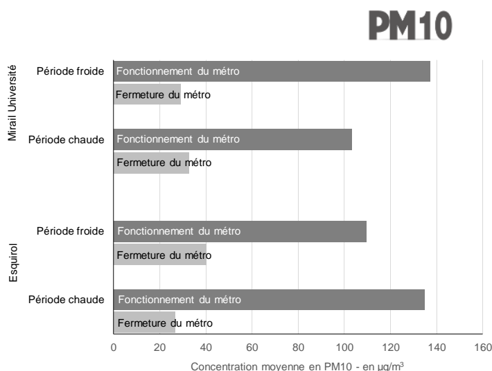
Graphe 4 : Niveaux en PARTICULES PM10 mesurés en période de fonctionnement et en période de fermeture du métro - stations de métro ESQUIROL et MIRAIL-UNIVERSITÉ .
