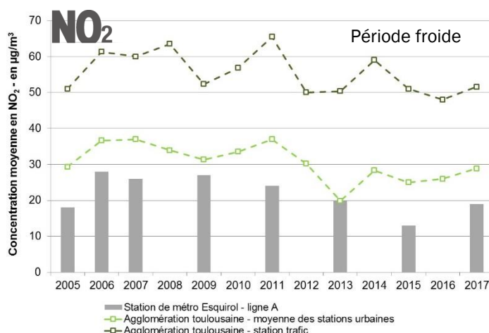
Graphie 21 : Évolution des concentrations moyennes en DIOXYDE D'AZOTE sur la période froide mesurées dans la station de métro ESQUIROL depuis 2005 et comparaison avec les concentrations rencontrées dans l'air ambiant extérieur.
