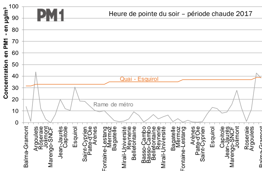
Graphe 19 : Évolution des concentrations en PM1 dans une rame de métro à l'heure de pointe du soir - PÉRIODE CHAUDE .
