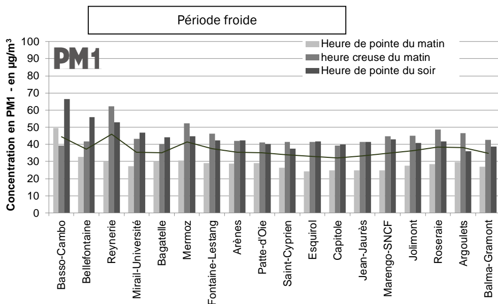
Graphe 20 : Évolution des concentrations en PARTICULES PM1 dans les rames de métro pendant la PÉRIODE FROIDE.
