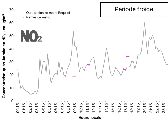
Graph 24 : Comparaison des concentrations en DIOXYDE D'AZOTE rencontrées dans les RAMES DE MÉTRO avec celles mesurées sur le quai de la station de métro ESQUIROL.
