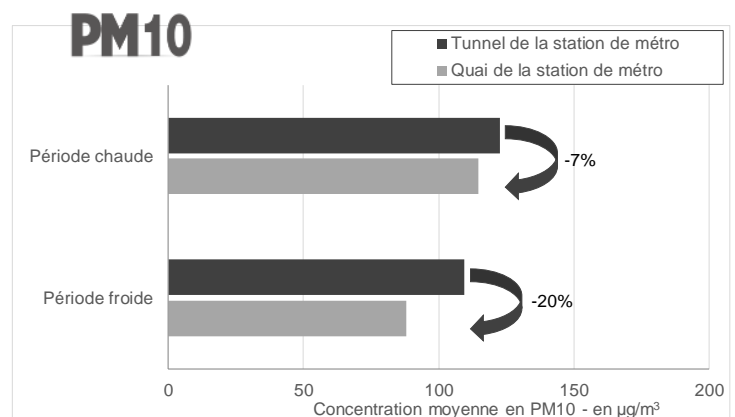
Graphe 16 : Niveaux en PARTICULES PM10 mesurés sur le QUAI dans le TUNNEL - station de ESQUIROL
