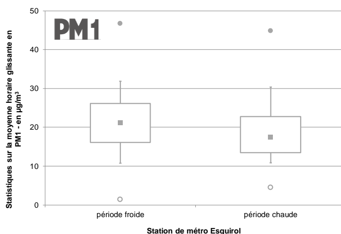
Graphe 9 : Répartition des concentrations horaires en PARTICULES PM1 mesurées dans la station de métro ESQUIROL.
