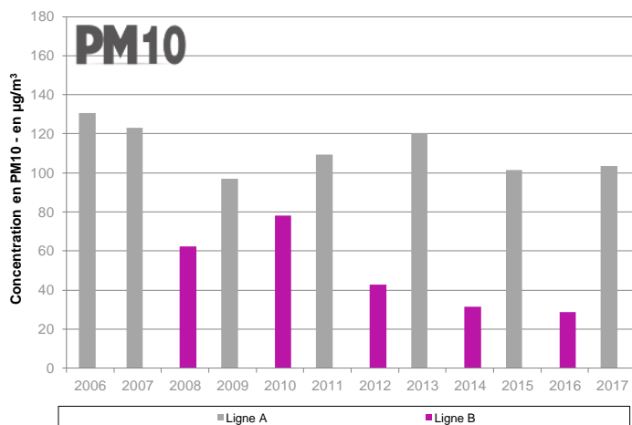
Graphe 12 : Évolution des niveaux en PM10 mesurées dans les deux lignes de métro depuis 2006.
