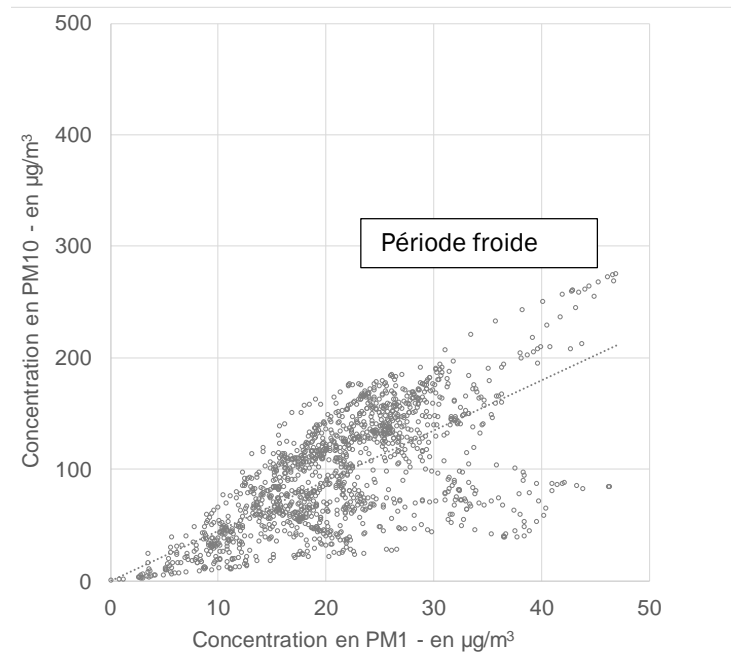
Graphe 15 : Évaluation de la relation éventuelle existant entre les niveaux de PARTICULES PM1 et PM10 mesurés sur le quai de la station de métro ESQUIROL
