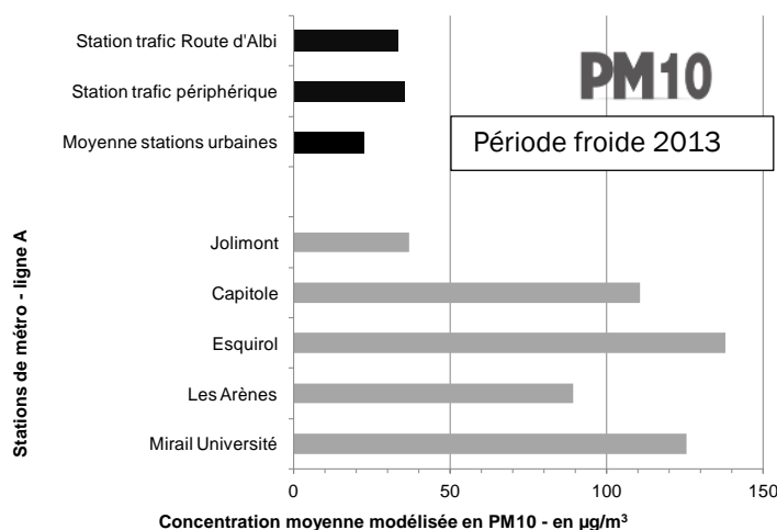
Graphe 1 : Concentration moyenne modélisée en PM10 dans les stations de métro et comparaison aux concentrations mesurées dans l'air ambiant extérieur - période froide 2013.
