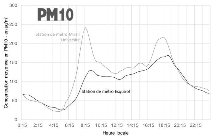
Graphe 6 : Comparaison des niveaux en PARTICULES PM10 mesurés sur les quais des DEUX STATIONS DE MÉTRO sur une journée moyenne en PÉRIODE FROIDE
