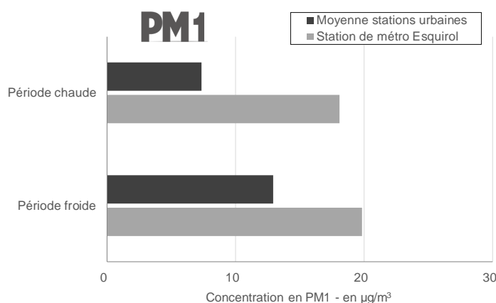
Graphique 13 : Concentration moyenne en PM1 dans les stations de métro et concentrations estimées dans l'air ambiant extérieur
