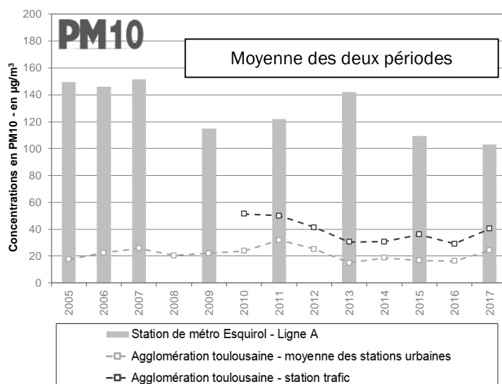
Graphe 11 : Evolution des concentrations en PM10 mesurées sur le quai de la station de métro ESQUIROL en MOYENNE SUR LES DEUX CAMPAGNES DE MESURES depuis 2005 et comparaison avec les concentrations rencontrées dans l'air ambiant.
