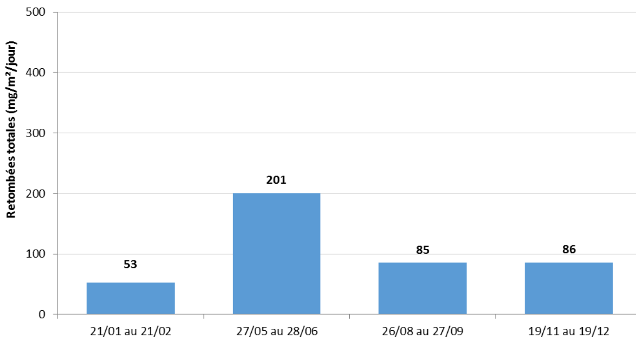
Suivi des retombées totales en 2019 – point de mesure BOR 1 (type a)
