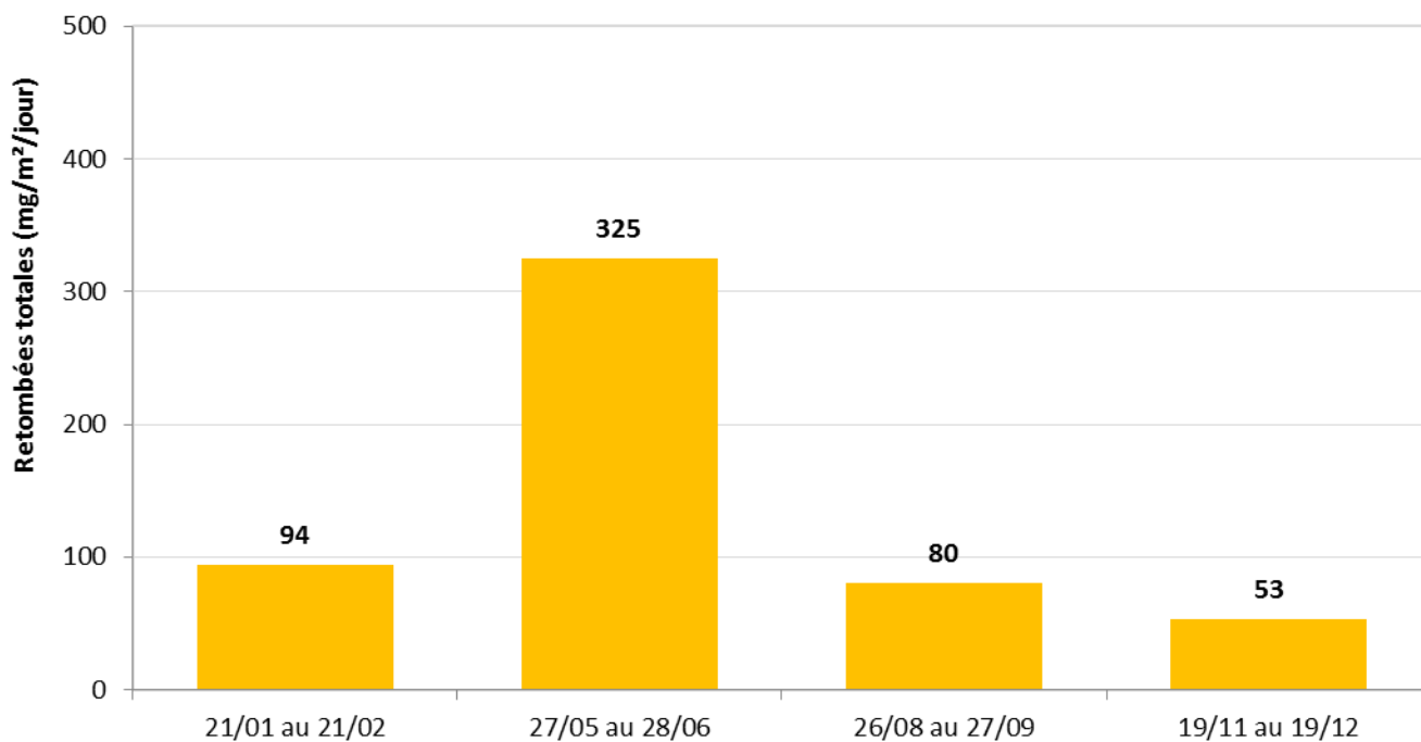
Suivi des retombées totales en 2019 – point de mesure BOR 3 (type b)
