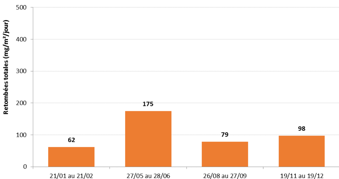
Suivi des retombées totales en 2019 – point de mesure BOR 2 (type c)
