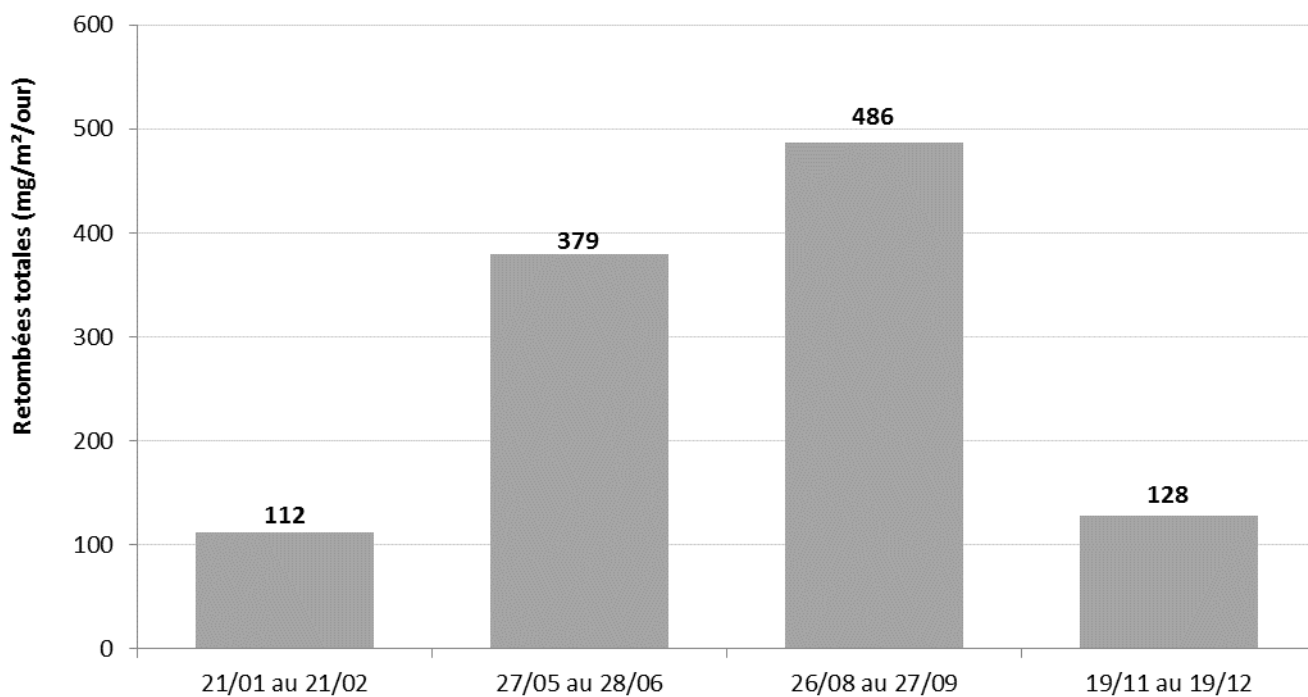
Suivi des retombées totales en 2019 – point de mesure BOR 4 (type c)
