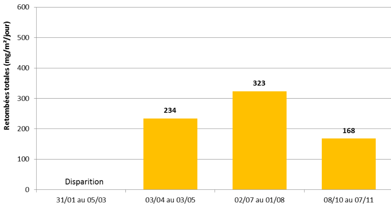
Suivi des retombées totales en 2019 – point de mesure PZ 5
