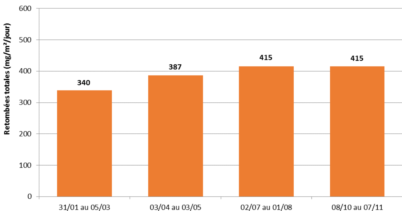
Suivi des retombées totales en 2019 – point de mesure PZ 2 (type c)
