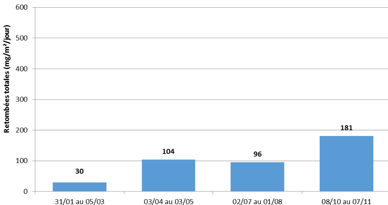
Suivi des retombées totales en 2019 – point de mesure PZ 1 (type a)
