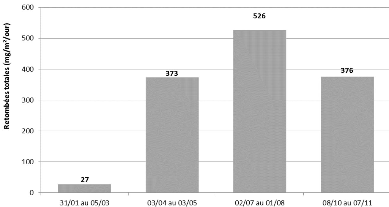
Suivi des retombées totales en 2019 – point de mesure PZ 3 (type c)
