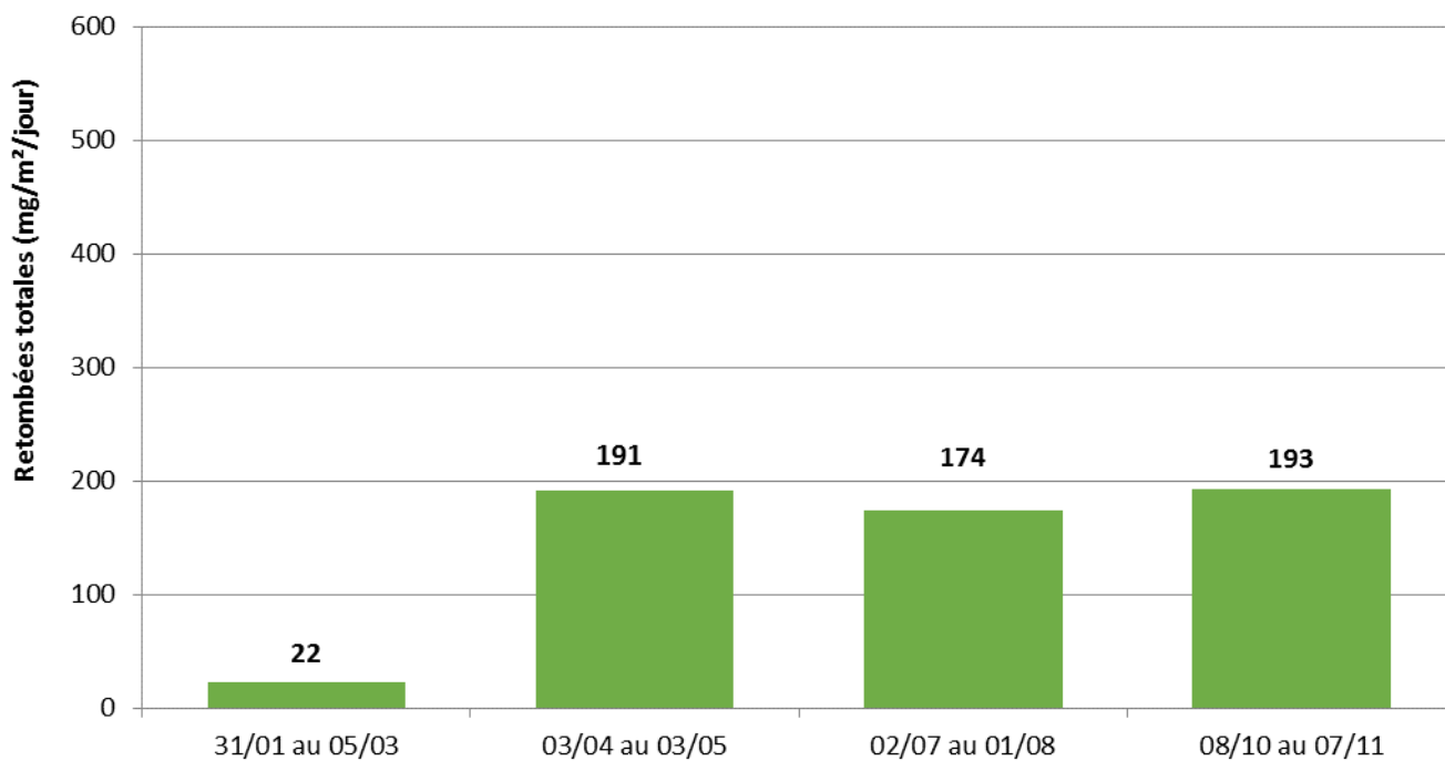
Suivi des retombées totales en 2019 – point de mesure PZ 4 (type b)
