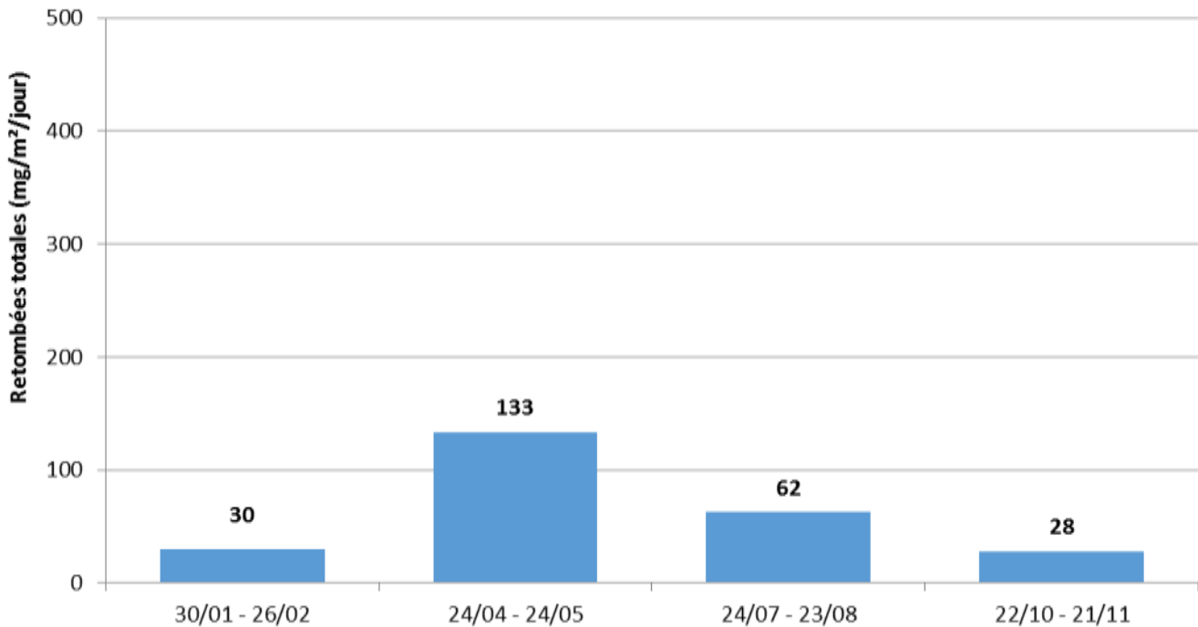
Suivi des retombées totales en 2019 – point de mesure LU 1 (type a)
