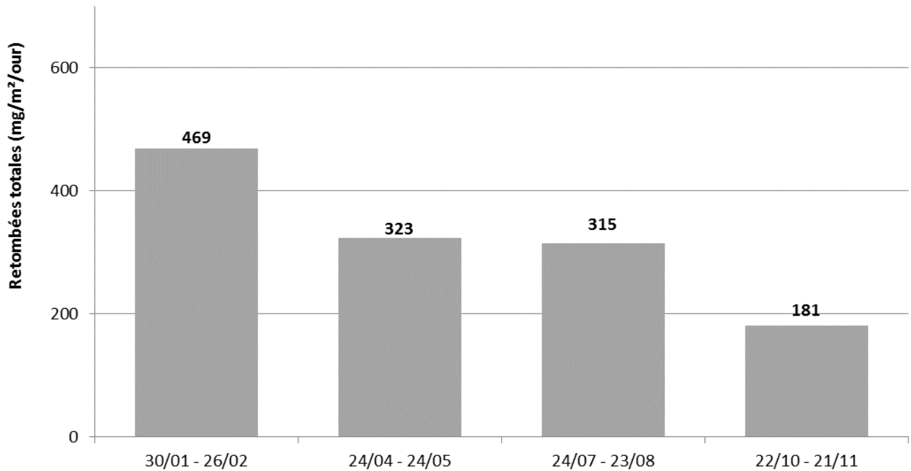
Suivi des retombées totales en 2019 – point de mesure LU 3 (type c)
