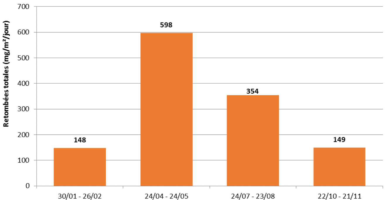
Suivi des retombées totales en 2019 – point de mesure LU 2 (type c)
