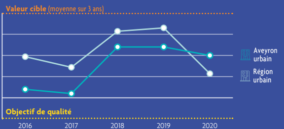
Évolution pluriannuelle O 3 Nombre de jours dépassant 120 µg/m 3 en moyenne glissante sur 8 heures.
