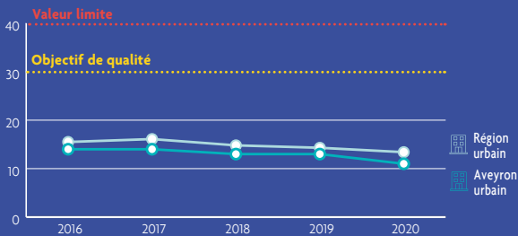
Évolution pluriannuelle PM10 Concentrations moyennes annuelles (µg/m 3 )
