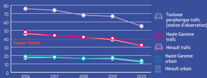
Évolution pluriannuelle NO 2 Concentrations moyennes annuelles (µg/m 3 )
