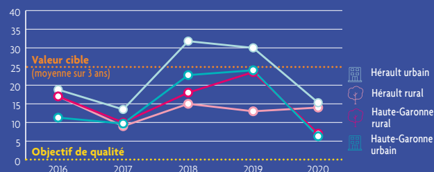
Évolution pluriannuelle O 3
