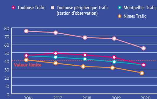
En proximité du trafic routier Concentration en µg/m³
