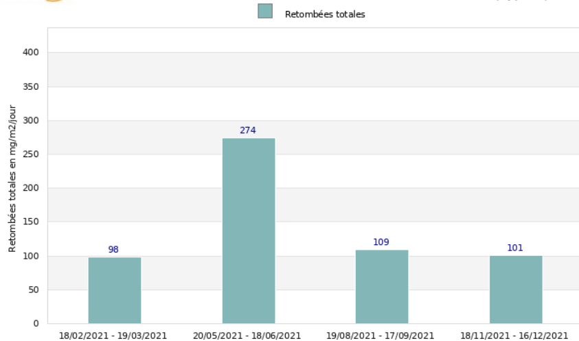
©Atmo-Occitanie Atmo OCCITANIE Site de Bordeneuve - Société Terreal Suivi des retombées totales en 2021 - Point de mesure BOR4 (Type c)
