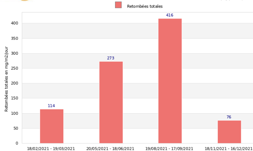
©Atmo-Occitanie Atmo OCCITANIE Site de Bordeneuve - Société Terreal Suivi des retombées totales en 2021 - Point de mesure BOR3 (Type b)
