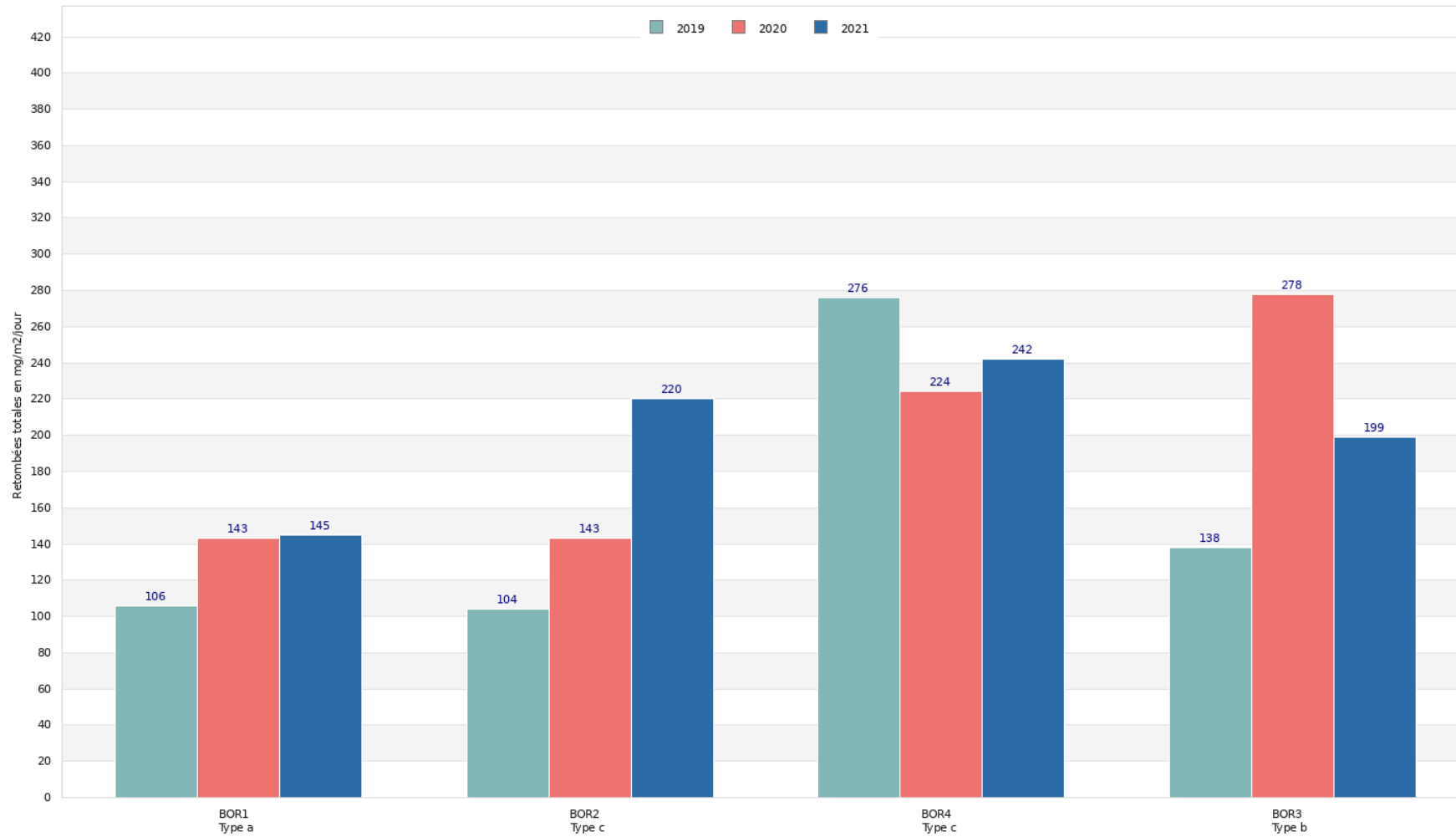
Site de Bordeneuve - Société Terreal Moyenne des retombées totales, évolution des moyennes annuelles depuis 2019
