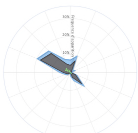
Rose des vents du 18/11/2021 au 16/12/2021
