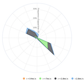
Rose des vents du 18/02/2021 au 19/03/2021
