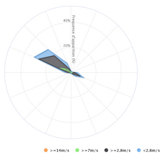
Rose des vents du 18/11/2021 au 16/12/2021
