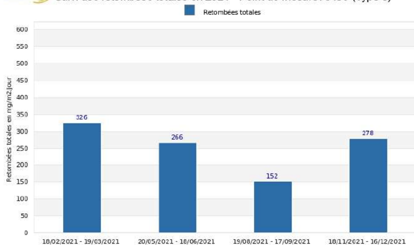
©Atmo-Occitanie Atmo OCCITANIE Site de La Caunette - Société Aude Agregats Suivi des retombées totales en 2021 - Point de mesure AAC3 (Type c)
