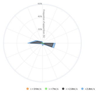
Rose des vents du 02/02/2021 au 06/04/2021
