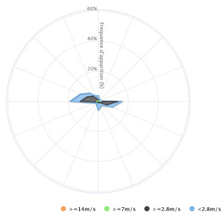
Rose des vents du 06/04/2021 au 04/06/2021
