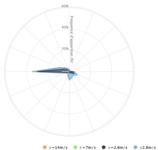
Rose des vents du 03/12/2020 au 02/02/2021
