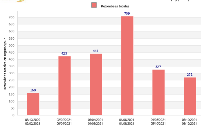
Site de Saverdun - CMGO Suivi des retombées totales en 2021 - Point de mesure X4 (Type c)
