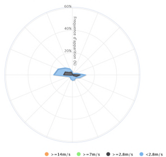
Rose des vents du 04/08/2021 au 05/10/2021
