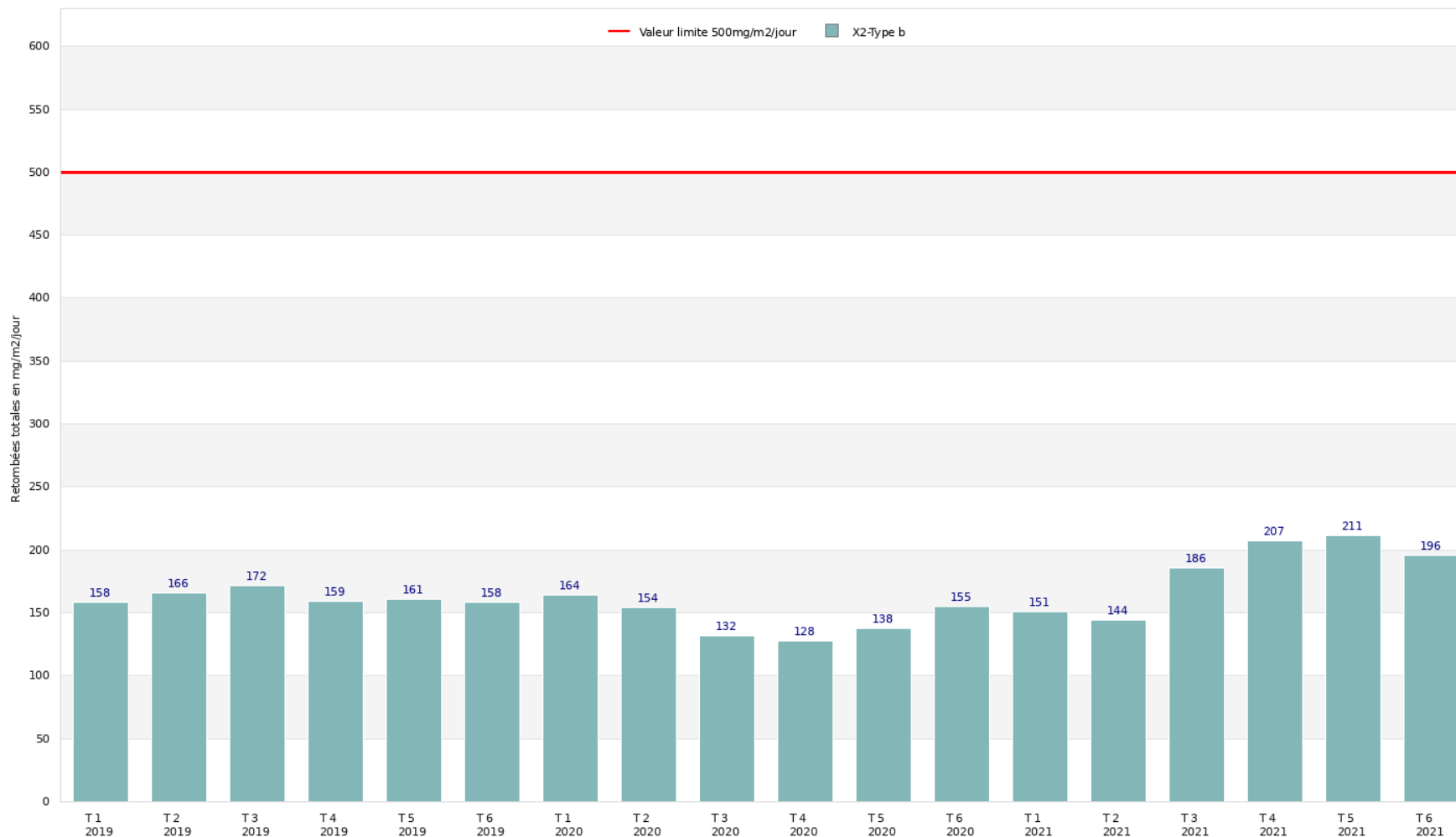
Site de Saverdun - CMGO Moyenne des retombées totales, évolution des moyennes glissantes
