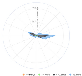
Rose des vents du 02/02/2021 au 04/03/2021
