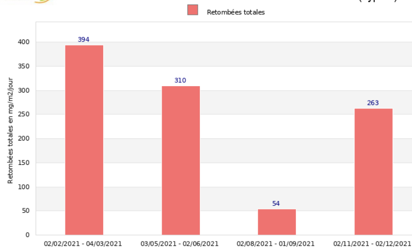
©Atmo-Occitanie Atmo OCCITANIE Site de Saint Arnac & Lansac - Société Imerys Suivi des retombées totales en 2021 - Point de mesure LAN 2 (Type b)
