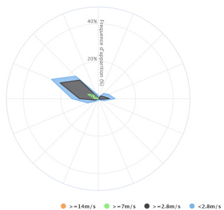
Rose des vents du 03/05/2021 au 02/06/2021
