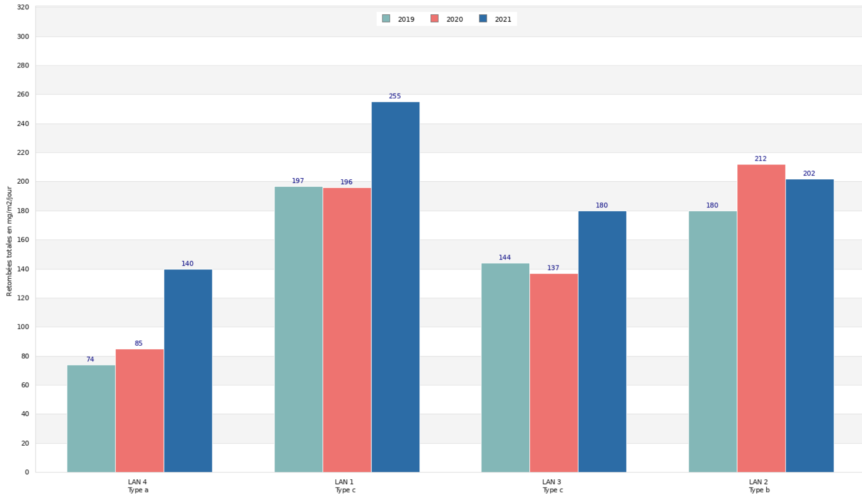
Site de Saint Arnac & Lansac - Société Imerys Moyenne des retombées totales, évolution des moyennes annuelles
