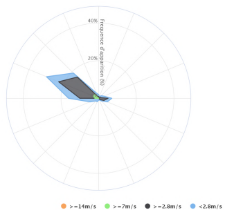
Rose des vents du 02/08/2021 au 01/09/2021
