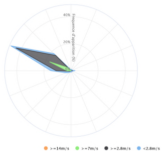
Rose des vents du 02/11/2021 au 02/12/2021
