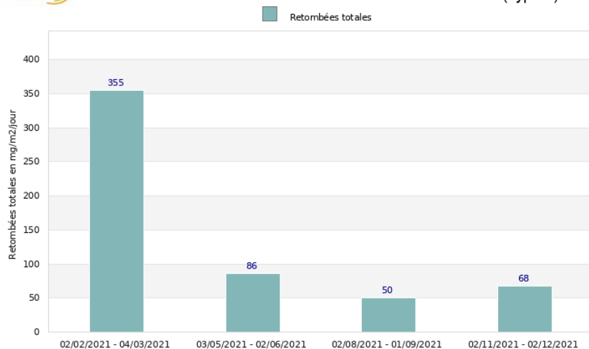
©Atmo-Occitanie Atmo OCCITANIE Site de Saint Arnac & Lansac - Société Imerys Suivi des retombées totales en 2021 - Point de mesure LAN 3 (Type c)
