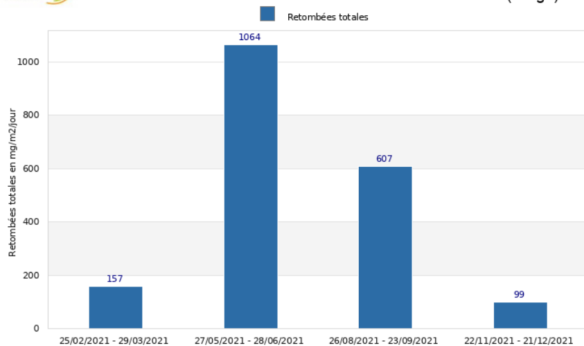
©Atmo-Occitanie Atmo OCCITANIE Site de St Laurent la Verne - Société Les Calcaires du Gard Suivi des retombées totales en 2021 - Point de mesure VERN 1 (Jauge)
