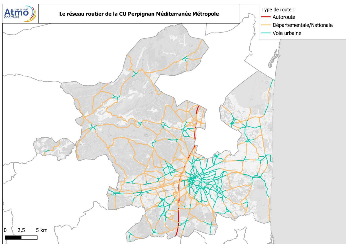
Répartition des émissions polluantes associées au trafic routier et des kilomètres parcourus sur le territoire par type de voies en 2019
