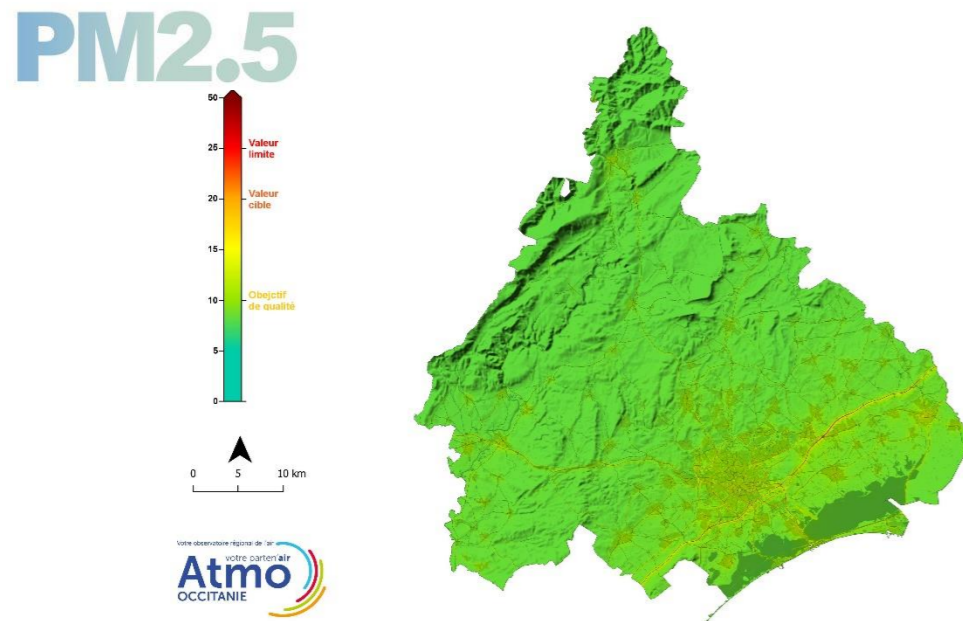
Concentrations moyennes annuelles en particules PM 2,5 – Territoire du PPA – année 2018
