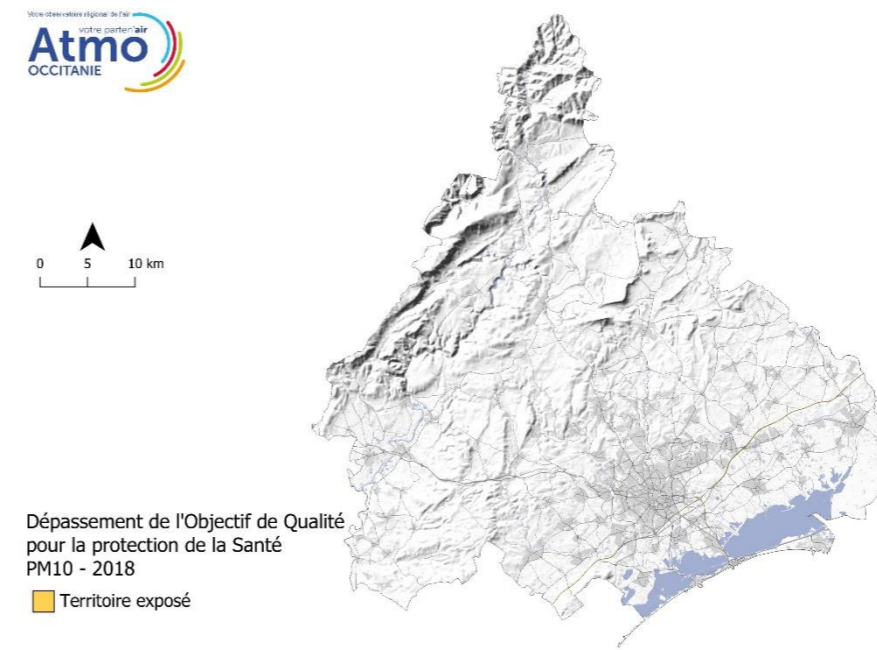
Exposition à l'objectif de qualité des particules PM 10 - Territoire du PPA – année 2018
