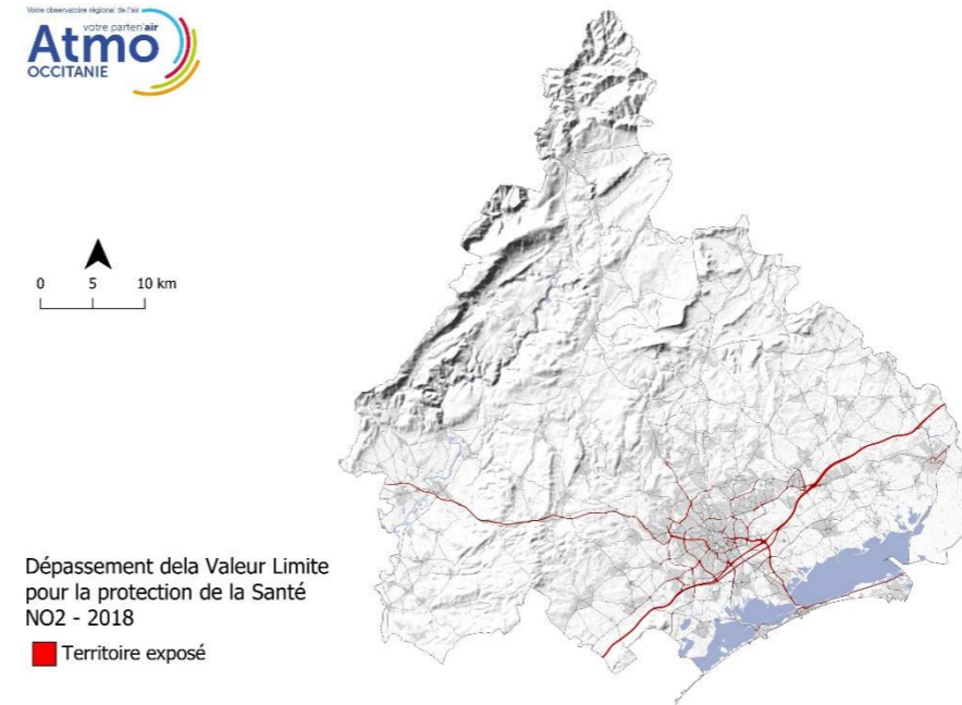
Exposition chronique au dioxyde d'azote - Territoire du PPA –année 2018 a
