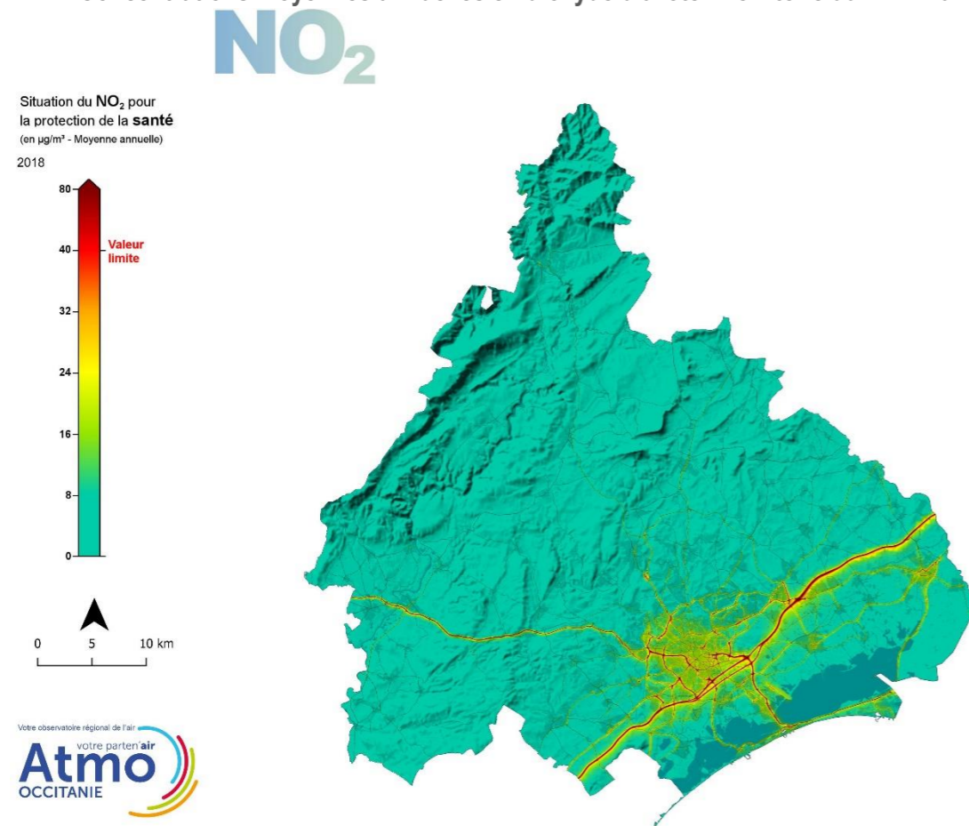
Concentrations moyennes annuelles en dioxyde d'azote - Territoire du PPA – année 2018
