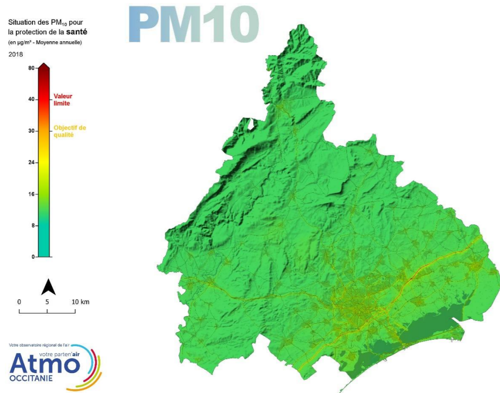
Concentrations moyennes annuelles en particules PM 10 – Territoire du PPA – année 2018
