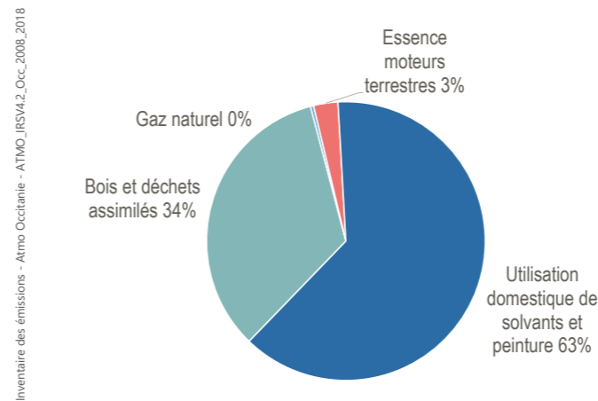
Type d'émissions résidentielles de Composés Organiques Volatils Non Méthaniques - Territoire du PPA –année 2018-
