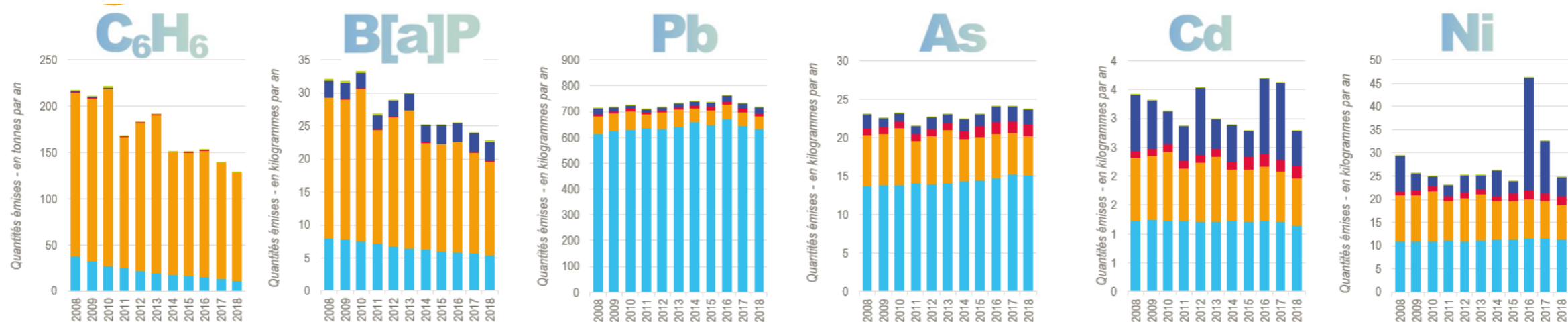
Évolution des contributions sectorielles aux émissions polluantes - Territoire du PPA – années 2008 à 2018 –
