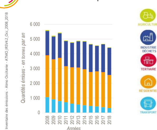
Évolution des contributions sectorielles aux émissions de Composés Organiques Volatils Non Méthaniques - Territoire du PPA – années 2008 à 2018 –
