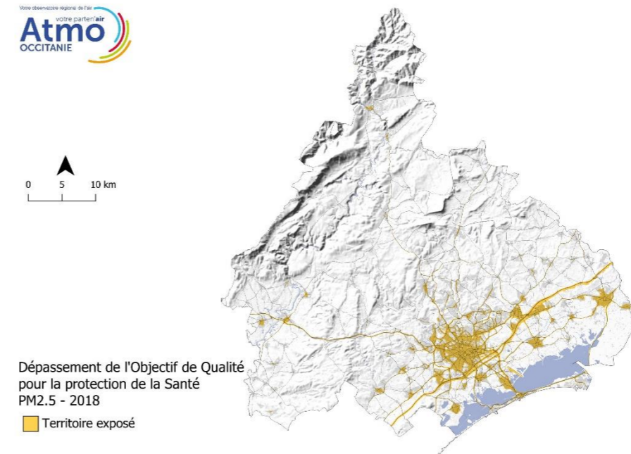
Exposition à l'objectif de qualité des particules PM 2,5 - Territoire du PPA – année 2018
