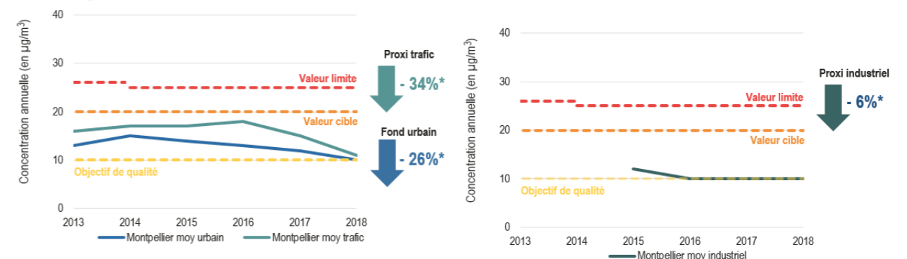
Évolution pluriannuelle des concentrations - Particules PM 2,5 - Territoire du PPA montpelliérain
