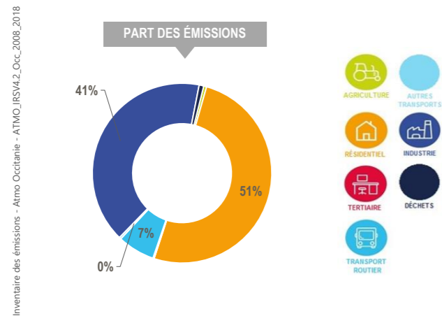
Contribution sectorielle aux émissions de Composés Organiques Volatils Non Méthaniques - Territoire du PPA –année 2018-
