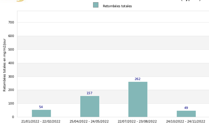
©Atmo-Occitanie Atmo OCCITANIE Site de St Laurent la Vernede - Société Les Calcaires du Gard Suivi des retombées totales en 2022 - Point de mesure VERN 1 (Jauge)
