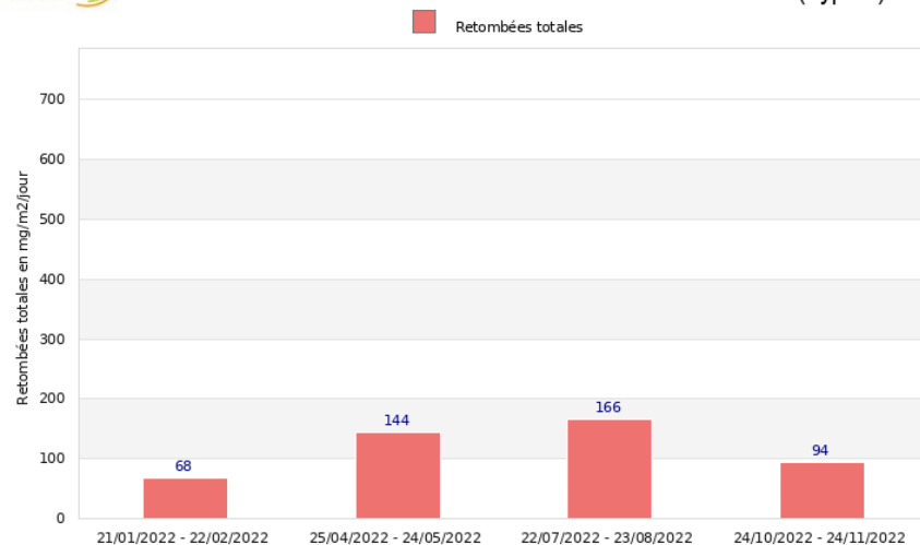
©Atmo-Occitanie Atmo OCCITANIE Site de St Laurent la Vernede - Société Les Calcaires du Gard Suivi des retombées totales en 2022 - Point de mesure VERN 3 (Jauge)
