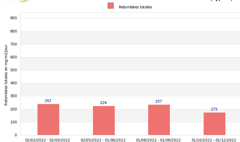
Site de Caves - Société Domitia Granulats Suivi des retombées totales en 2022 - Point de mesure CAVES 3 (Type b)
