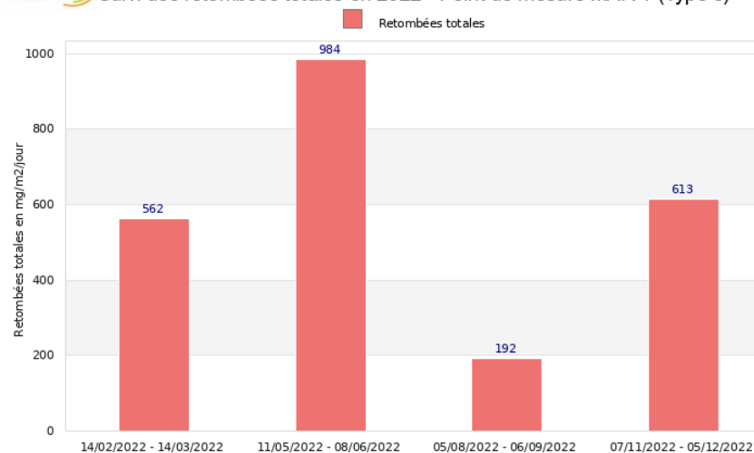
Site de Maraussan - Sablière du littoral Suivi des retombées totales en 2022 - Point de mesure MAR 3 (Type c)
