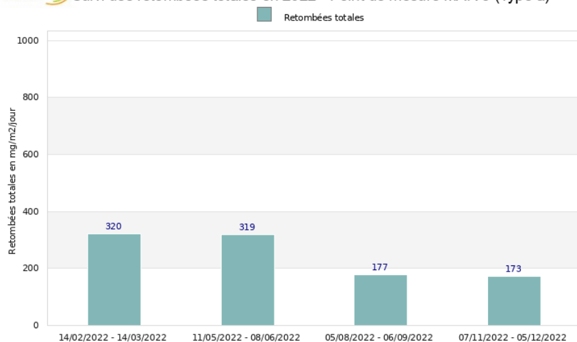
Site de Maraussan - Sablière du littoral Suivi des retombées totales en 2022 - Point de mesure MAR 2 (Type c)
