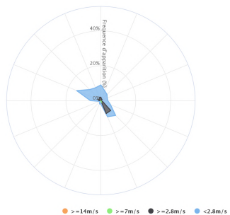
Rose des vents du 14/02/2022 au 14/03/2022
