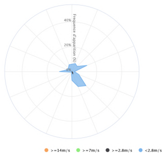
Rose des vents du 11/05/2022 au 08/06/2022
