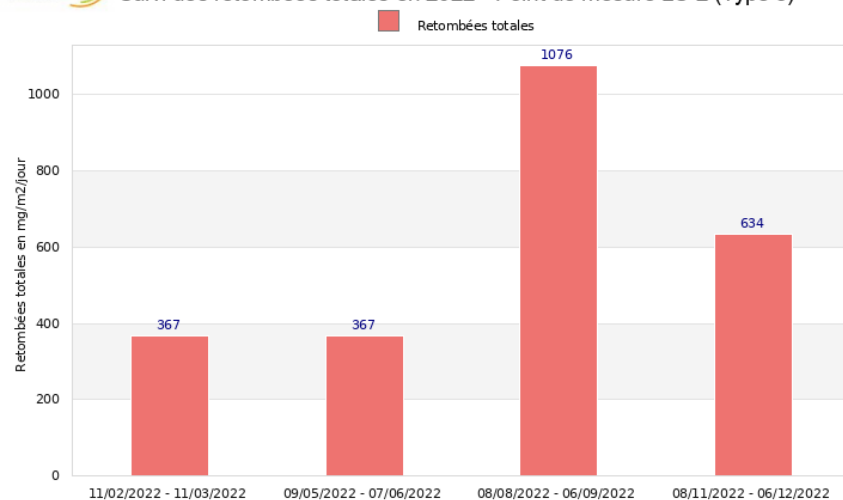
Site de Saturargues - Société LRM Suivi des retombées totales en 2022 - Point de mesure LU 2 (Type c)
