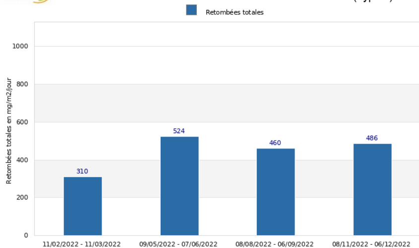
Site de Saturargues - Société LRM Suivi des retombées totales en 2022 - Point de mesure LU 3 (Type c)
