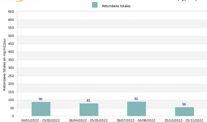
©Atmo-Occitanie Atmo OCCITANIE Site de Mas de Cournon - Société Biocama Suivi des retombées totales en 2022 - Point de mesure MAS 3 (Type c)
