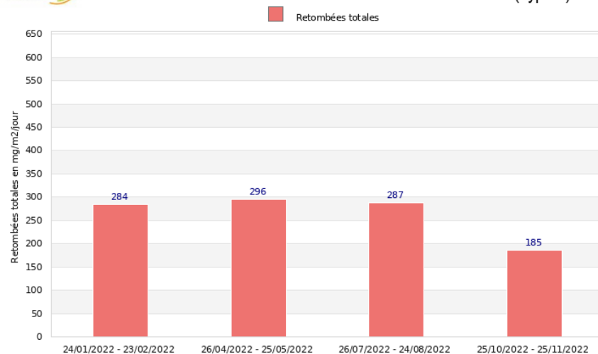
©Atmo-Occitanie Atmo OCCITANIE Site de Mas de Cournon - Société Biocama Suivi des retombées totales en 2022 - Point de mesure MAS 4 (Type b)
