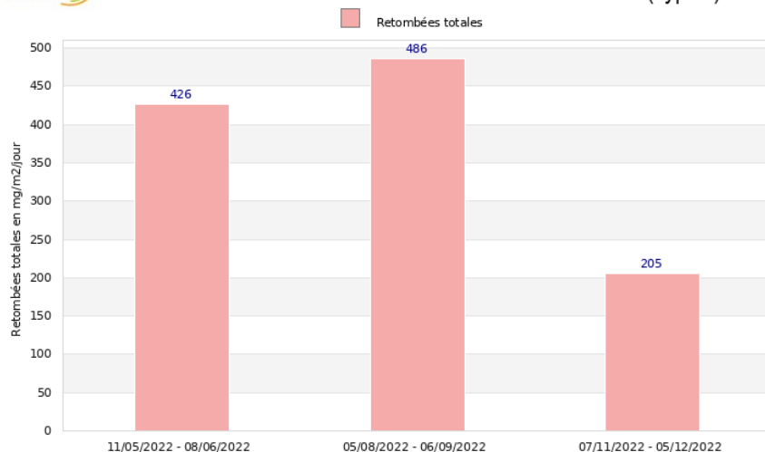
Site de Saint Pons - Société CMSE Suivi des retombées totales en 2022 - Point de mesure SP 5 (Type c)
