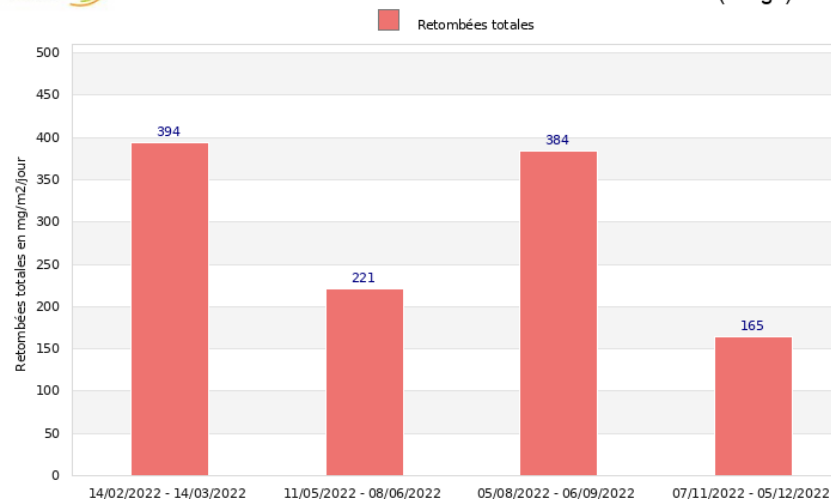
Site de Saint Pons - Société CMSE Suivi des retombées totales en 2022 - Point de mesure SP 4 (Jauge)
