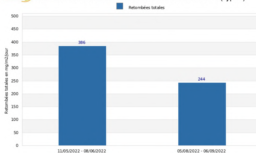
Site de Saint Pons - Société CMSE Suivi des retombées totales en 2022 - Point de mesure SP 1 (Type c)
