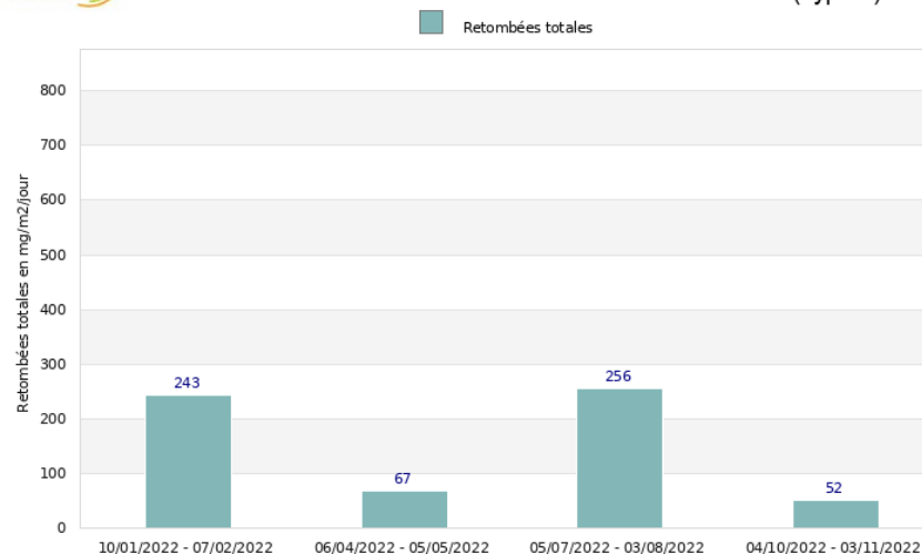
Site de Thuir - Société CMSE Suivi des retombées totales en 2022 - Point de mesure TH 4 (Type b)
