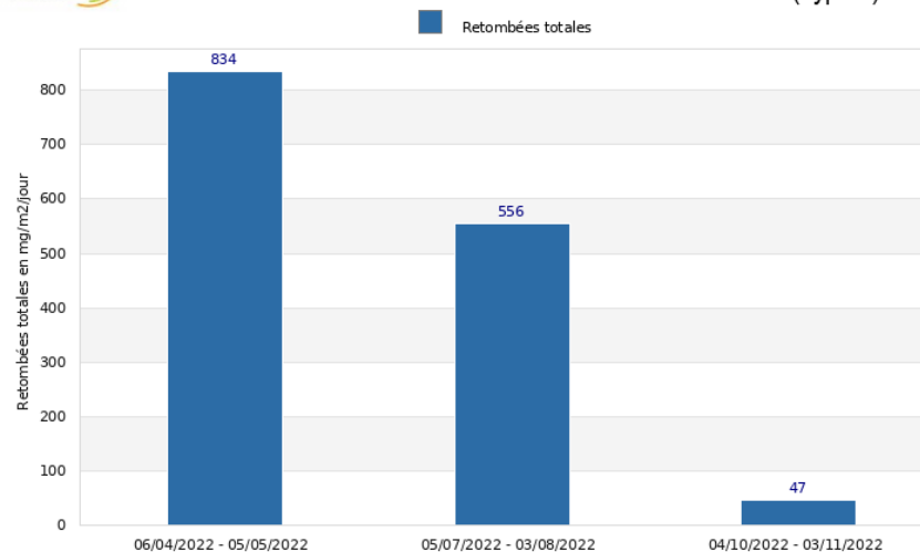
Site de Thuir - Société CMSE Suivi des retombées totales en 2022 - Point de mesure TH 3 (Type c)
