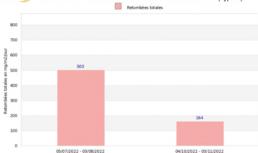
Site de Thuir - Société CMSE Suivi des retombées totales en 2022 - Point de mesure TH 2 (Type b)
