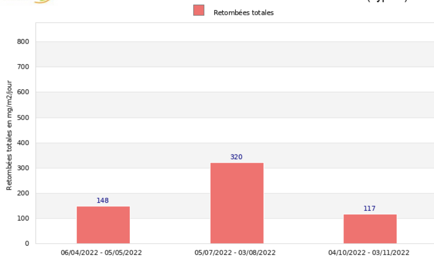
Site de Thuir - Société CMSE Suivi des retombées totales en 2022 - Point de mesure TH 1 (Type a)
