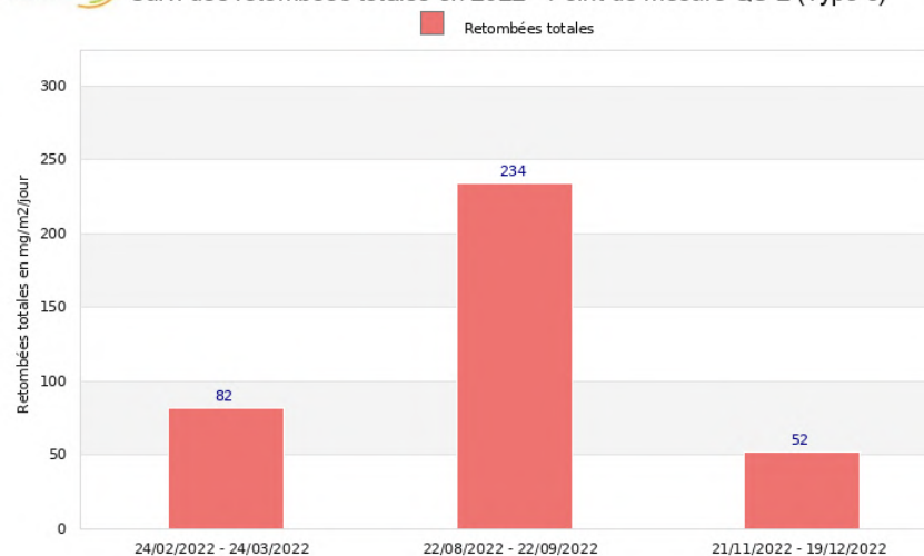
Atmo OCCITANIE Site de Quillan - Domitia Granulats Suivi des retombées totales en 2022 - Point de mesure QU 2 (Type c)
