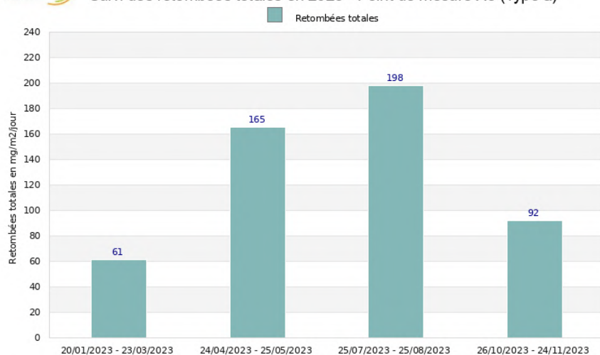
Site de Varilhes - CMGO Suivi des retombées totales en 2023 - Point de mesure X5 (Type a)
