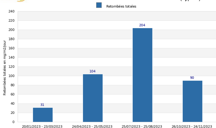
Site de Varilhes - CMGO Suivi des retombées totales en 2023 - Point de mesure R2 (Type b)
