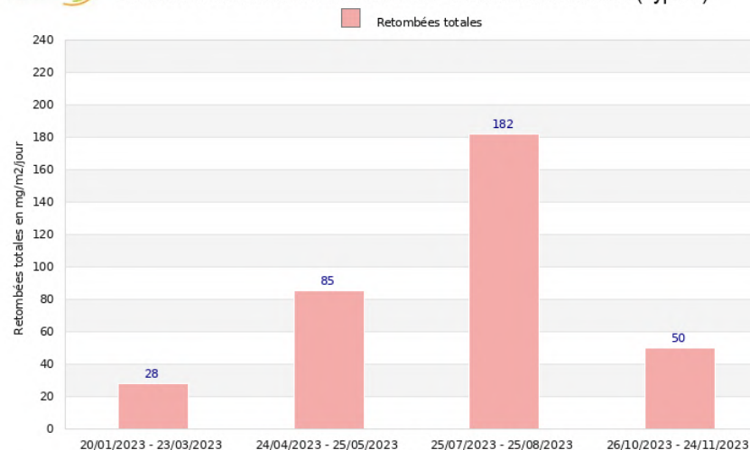
Site de Varilhes - CMGO Suivi des retombées totales en 2023 - Point de mesure R3 (Type b)
