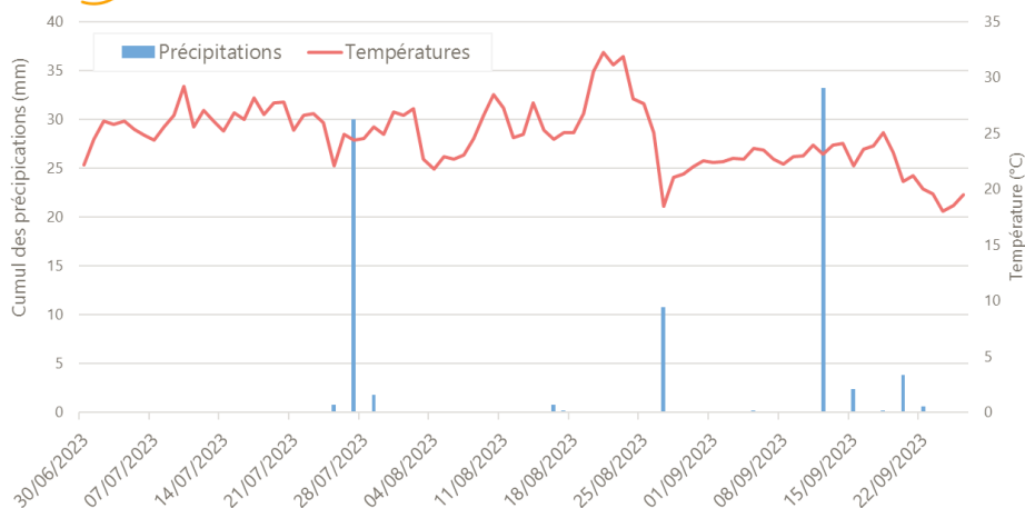
Evolution des températures et du cumul journalier des précipitations (Troisième trimestre 2023)
