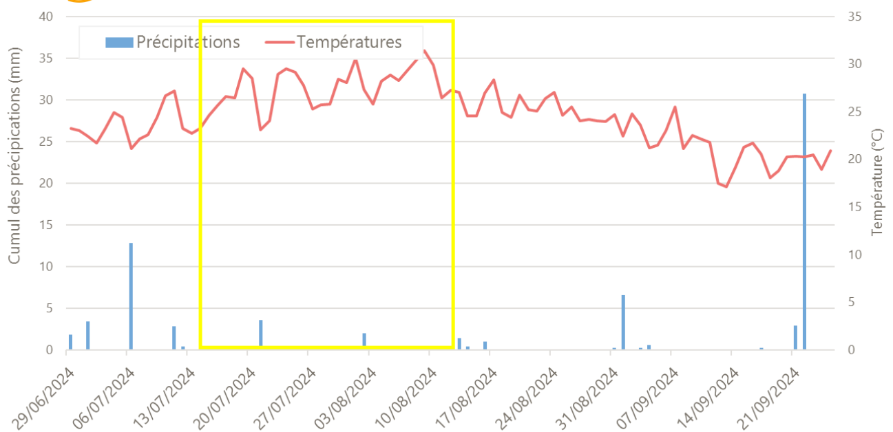
Evolution des températures et du cumul journalier des précipitations (Troisième trimestre 2024)
