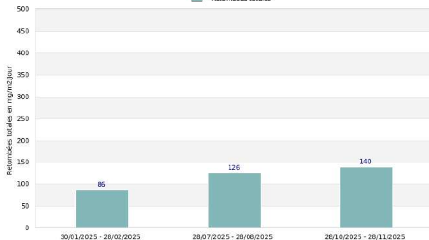
©Atmo-Occitanie Atmo OCCITANIE Site de Pouzilhac - Société RCI Suivi des retombées totales en 2025 - Point de mesure RCI 2 (Jauge)
