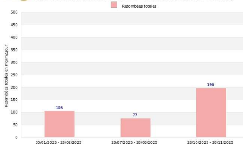
©Atmo-Occitanie Atmo OCCITANIE Site de Pouzilhac - Société RCI Suivi des retombées totales en 2025 - Point de mesure RCI 3 (Jauge)
