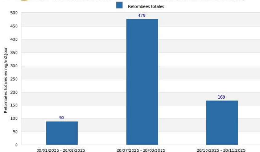
©Atmo-Occitanie Atmo OCCITANIE Site de Pouzilhac - Société RCI Suivi des retombées totales en 2025 - Point de mesure RCI 2 (Jauge)
