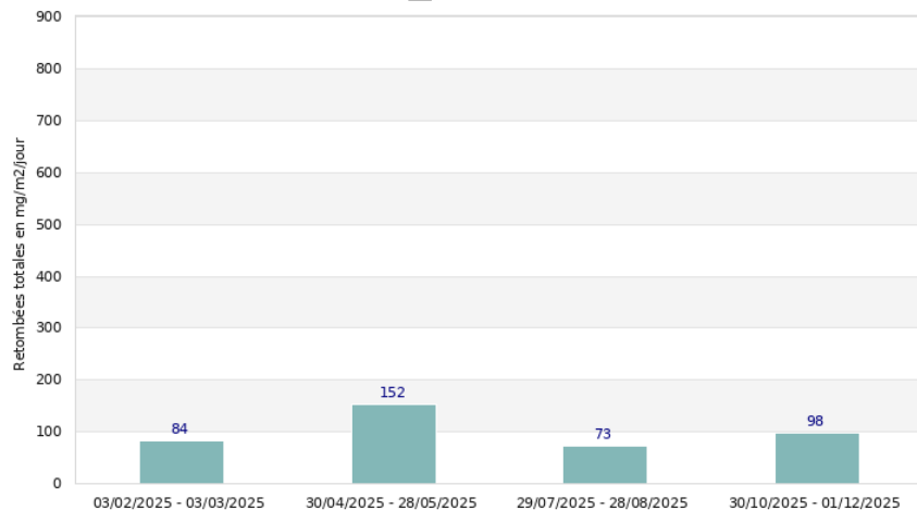
Atmo OCCITANIE Site de Port la Nouvelle carrière - Société Lafarge Ciments Suivi des retombées totales en 2025 - Point de mesure PLNC 5 (Type c)
