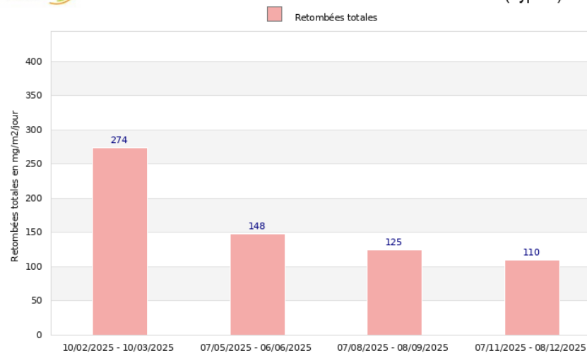
Site de Thoiras - Société Henry Leygue Suivi des retombées totales en 2025 - Point de mesure TO 3 (Type b)
