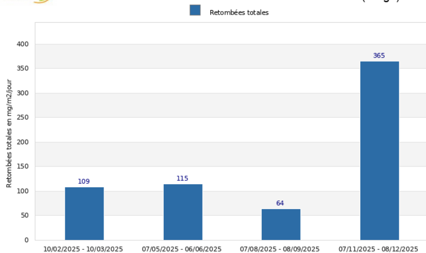
Site de Thoiras - Société Henry Leygue Suivi des retombées totales en 2025 - Point de mesure TO 4 (Jauge)
