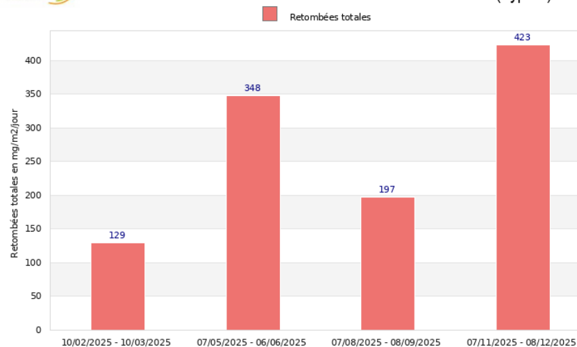
Site de Thoiras - Société Henry Leygue Suivi des retombées totales en 2025 - Point de mesure TO 5 (Type c)
