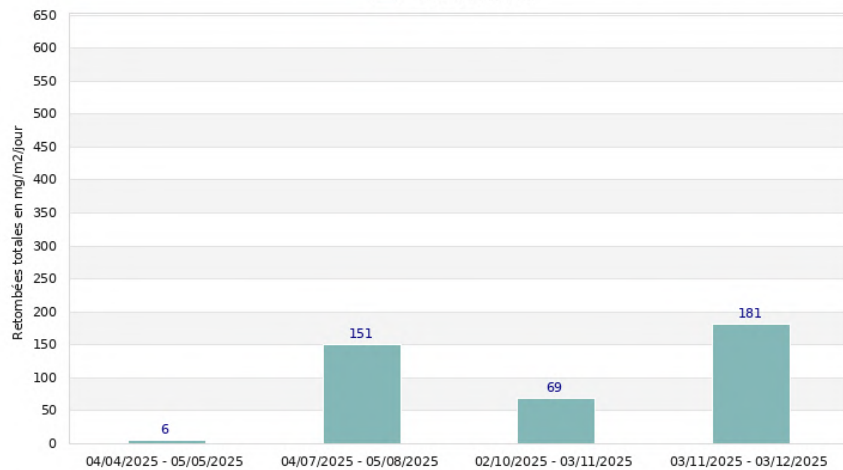
Atmo OCCITANIE Site de Les Bondons - Société SRC Suivi des retombées totales en 2025 - Point de mesure BON A (Type a)
