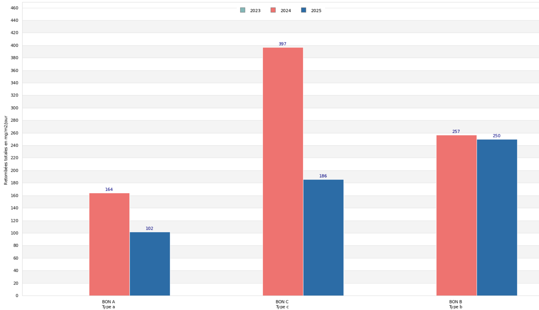
Site de Les Bondons - Société SRC Moyenne des retombées totales, évolution des moyennes annuelles
