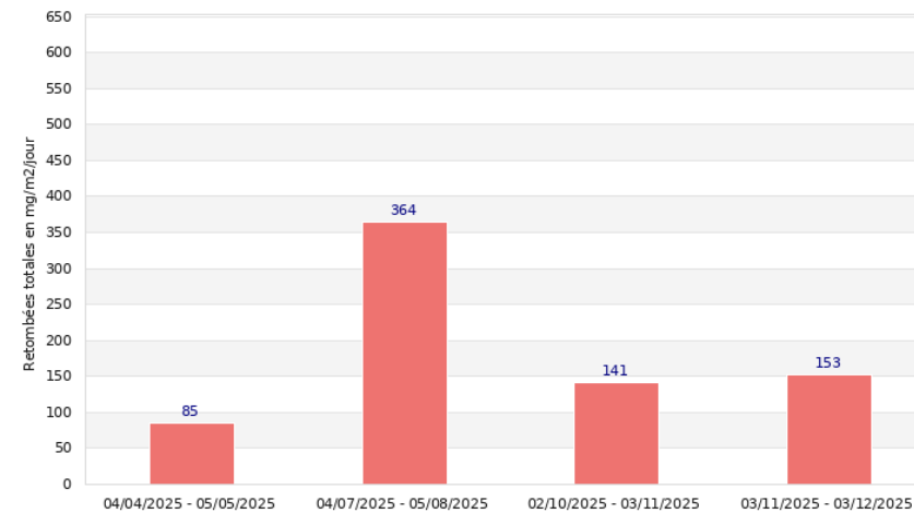
Atmo OCCITANIE Site de Les Bondons - Société SRC Suivi des retombées totales en 2025 - Point de mesure BON C (Type c)
