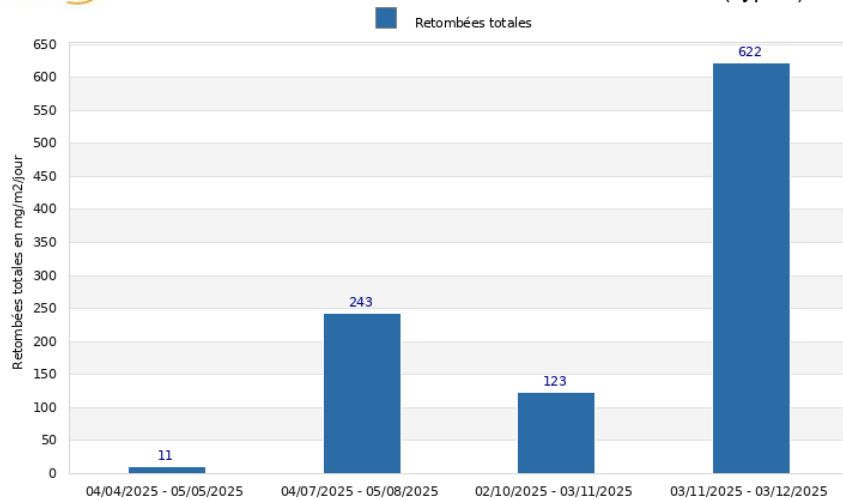
Atmo OCCITANIE Site de Les Bondons - Société SRC Suivi des retombées totales en 2025 - Point de mesure BON B (Type b)
